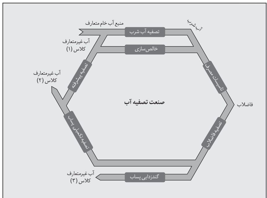
شکل شماره ۴-۷- گردش انسان ساخت آب برای استفاده دوباره ۲
