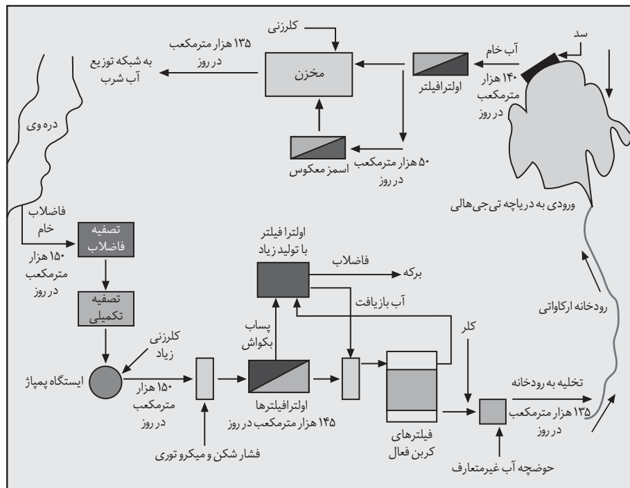
شکل شماره ۶-۲ - دیگرام پیشنهادی فرایند تصفیه برای فاز ۱ به ظرفیت ۱۳۵ هزار مترمکعب در روز
