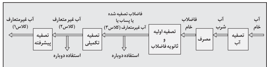
شکل شماره ۱-۱- دیاگرام کلی گردش آب در تاسیسات شهری
